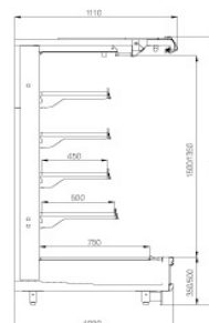
2.0m Height
